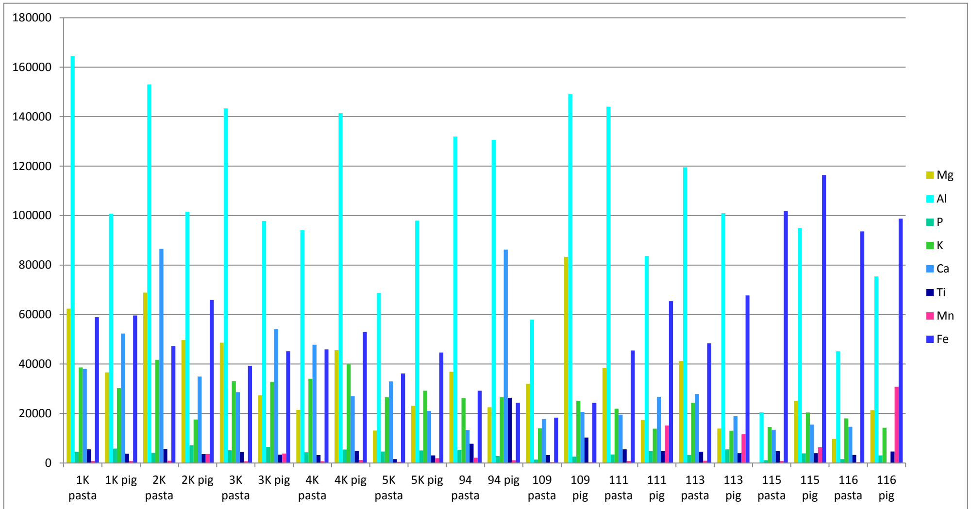
Gráfico N° 103 Composición química elemental de pigmentos
