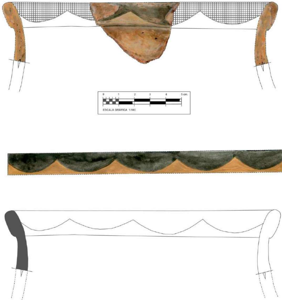
Figura N° 49.- Reconstrucción hipotética de un borde de un cántaro estilo killke
