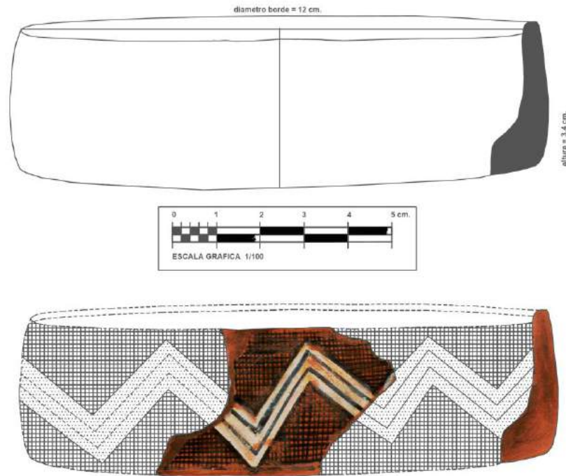
Figura N° 64.- Reconstrucción hipotética de una olla estilo Inka
