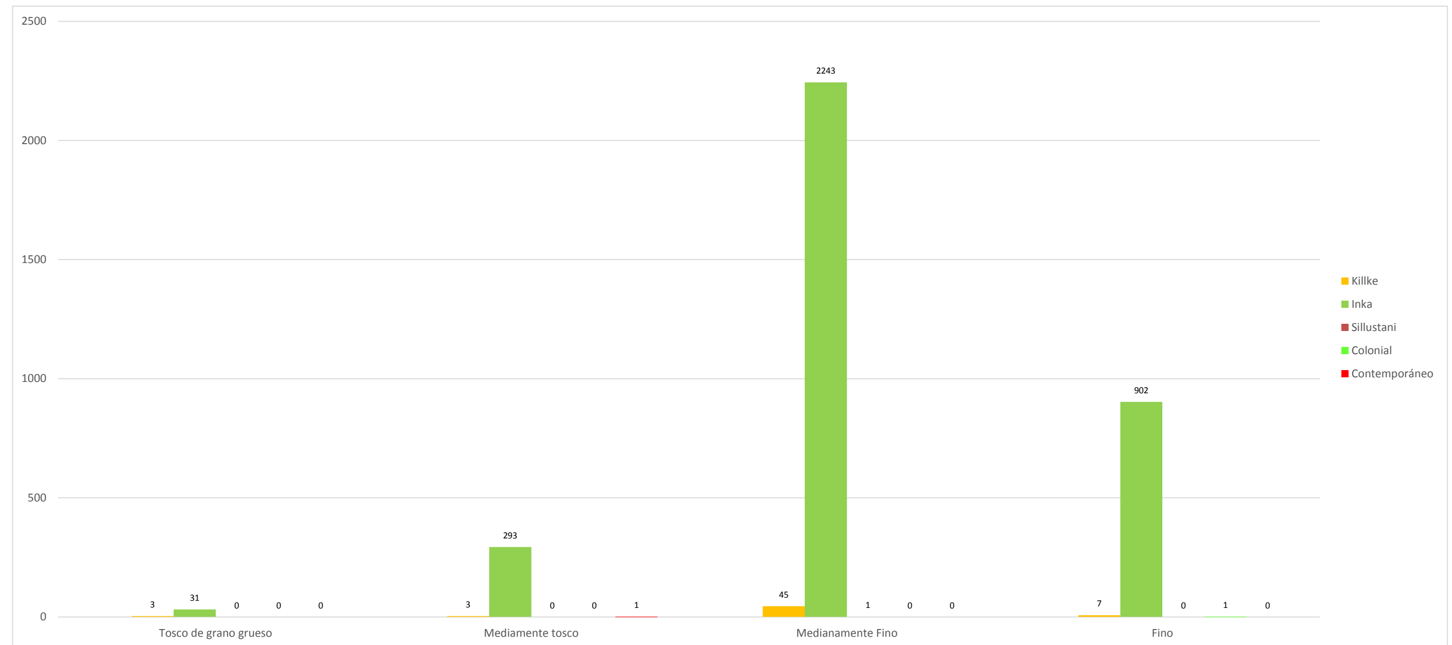
Gráfico N° 41.- Granulometría de los temperantes Fuente: Elaboración propia
