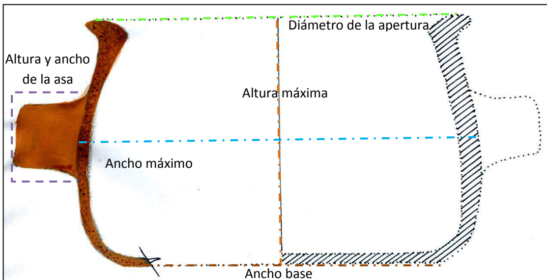
Figura N° 03: Medidas proporcionales entre altura, ancho, diámetro en una representación grafica técnica de una olla
