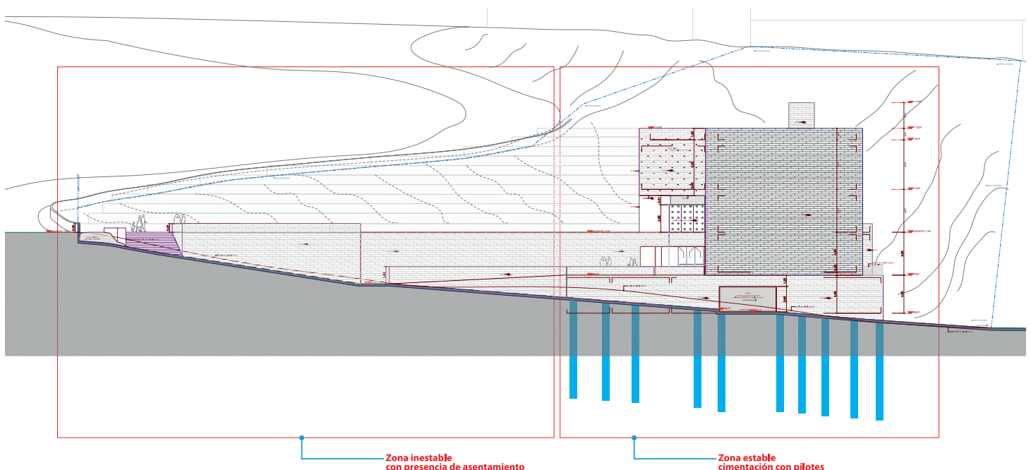
Imagen en elevación en donde se evidencia que el edificio principal, que se encuentra sobre pilotes, está estable; solo la explanada que, apoyada en terreno, presenta hundimiento.
