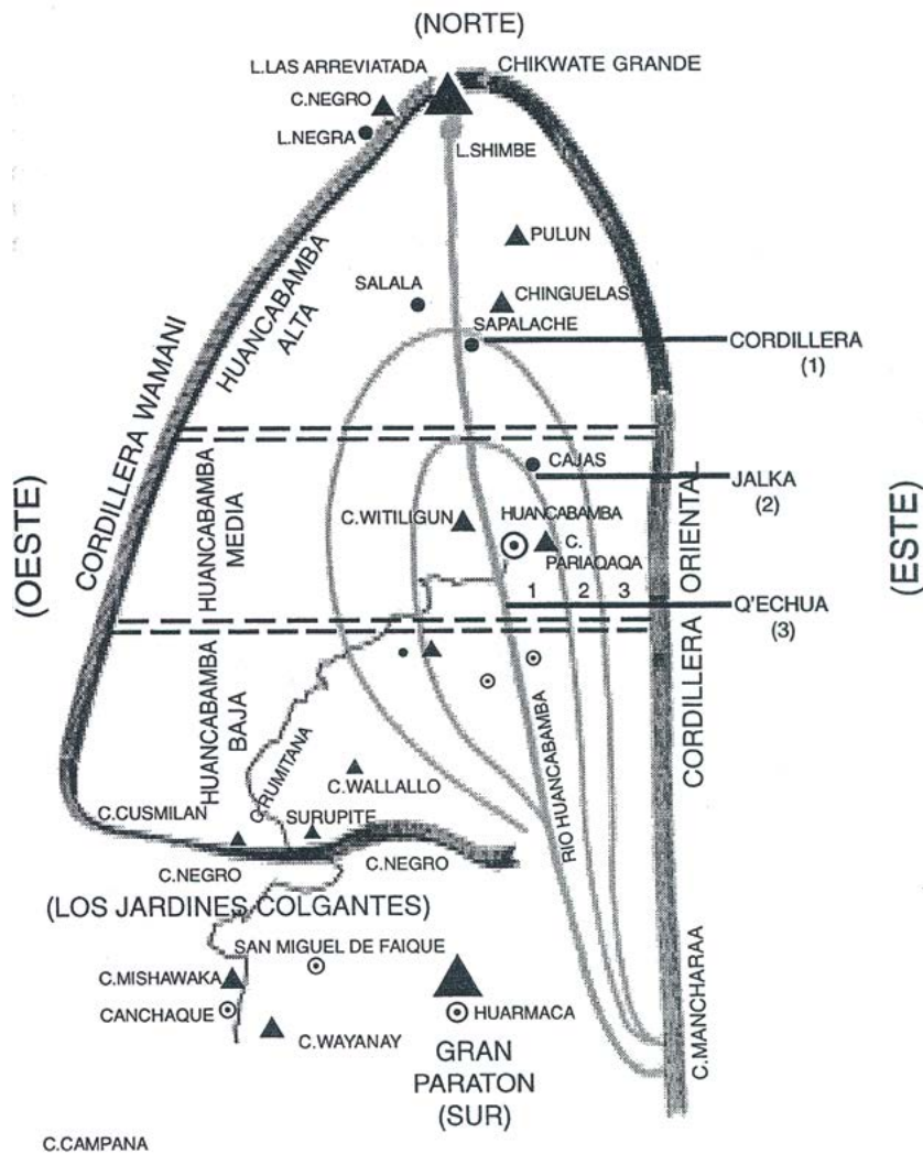
Esquema tentativo de la configuración geográfica de los pisos ecológicos de la cuenca del Huancabamba Fuente: (Arroyo 2004)
